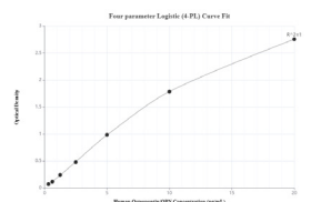
▲OPN/SPP1 重组抗体对 (MP00375-1) 的双抗夹心ELISA标准曲线
