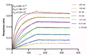
▲OPN/SPP1 重组捕获抗体 (83341-2-PBS) 的亲和力和动力学表征，亲和力常数为 0.468 nM
